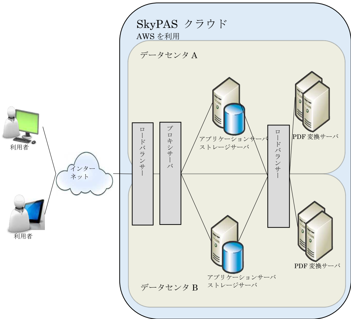
図 1システム概念図
